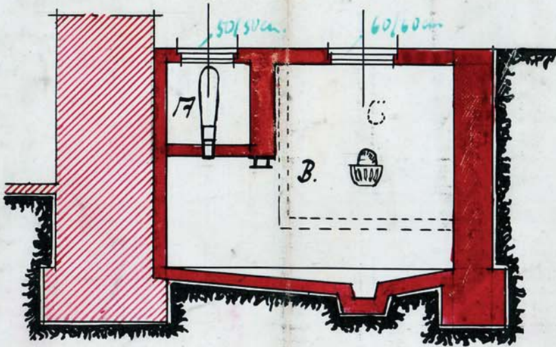
Schnitt durch die Closetgrube. M. = 1:50
